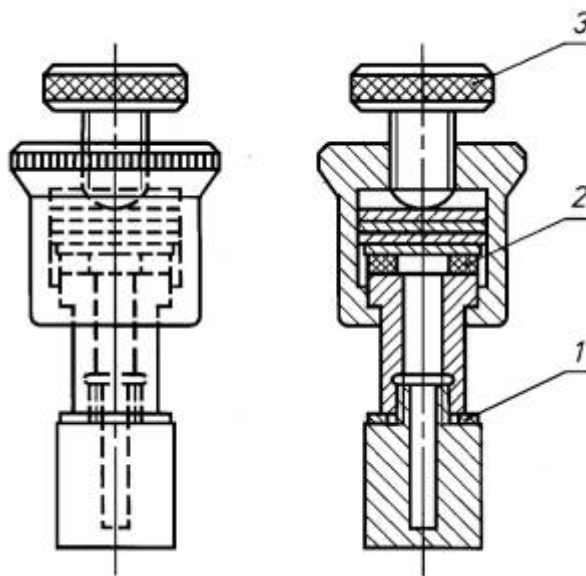
1 - металлическая прокладка; 2 - испытуемый образец; 3 - зажимной винт
