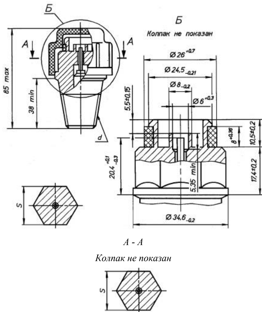
Рисунок 1 - Клапан
